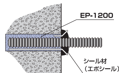
横向きアンカー施工例
